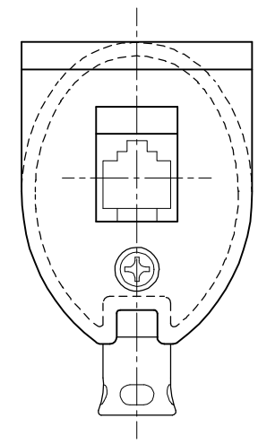
<A矢視 (側面図)>
